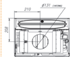
vista dall'alto C24
