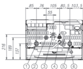
vista dal basso C-LOW NOx
