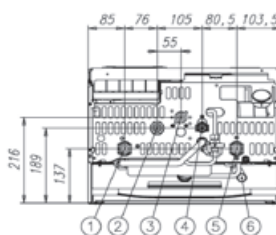
vista dal basso F-LOW NOx
