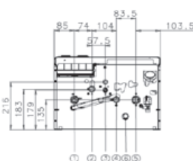
vista dal basso HF24-HF32
