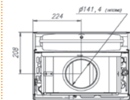
vista dall'alto C32
